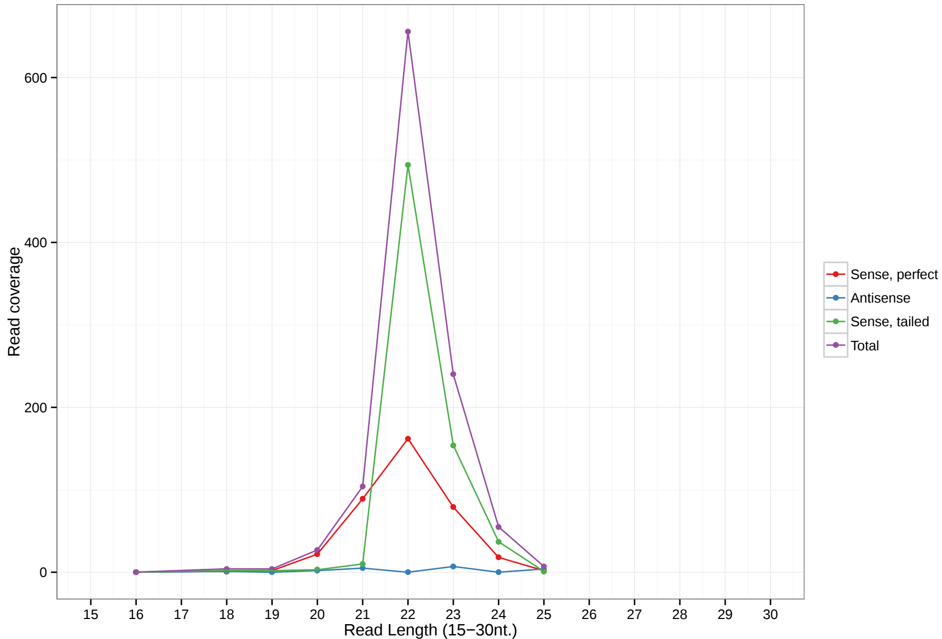
mmu-mir-7043
