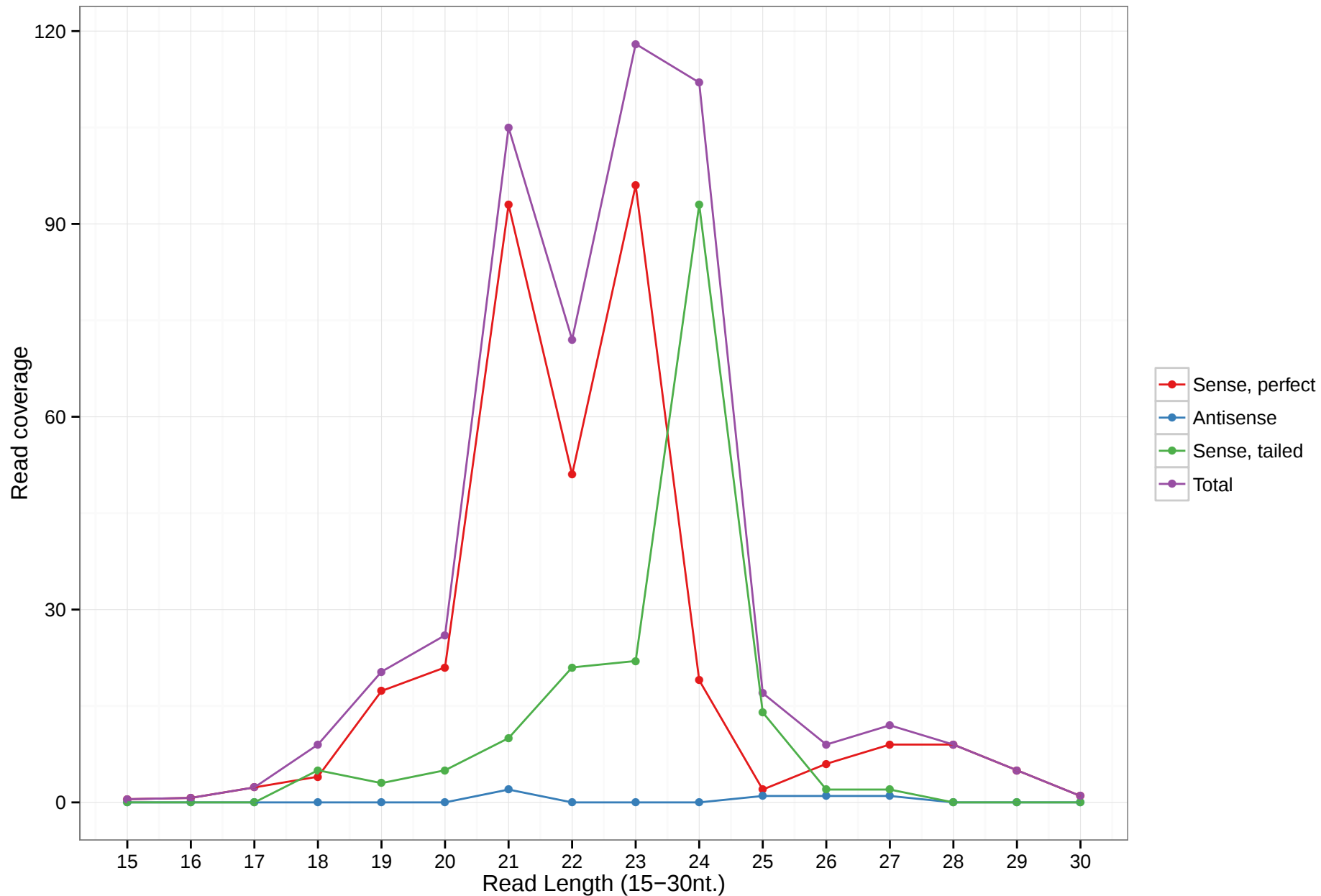
mmu-mir-7019
