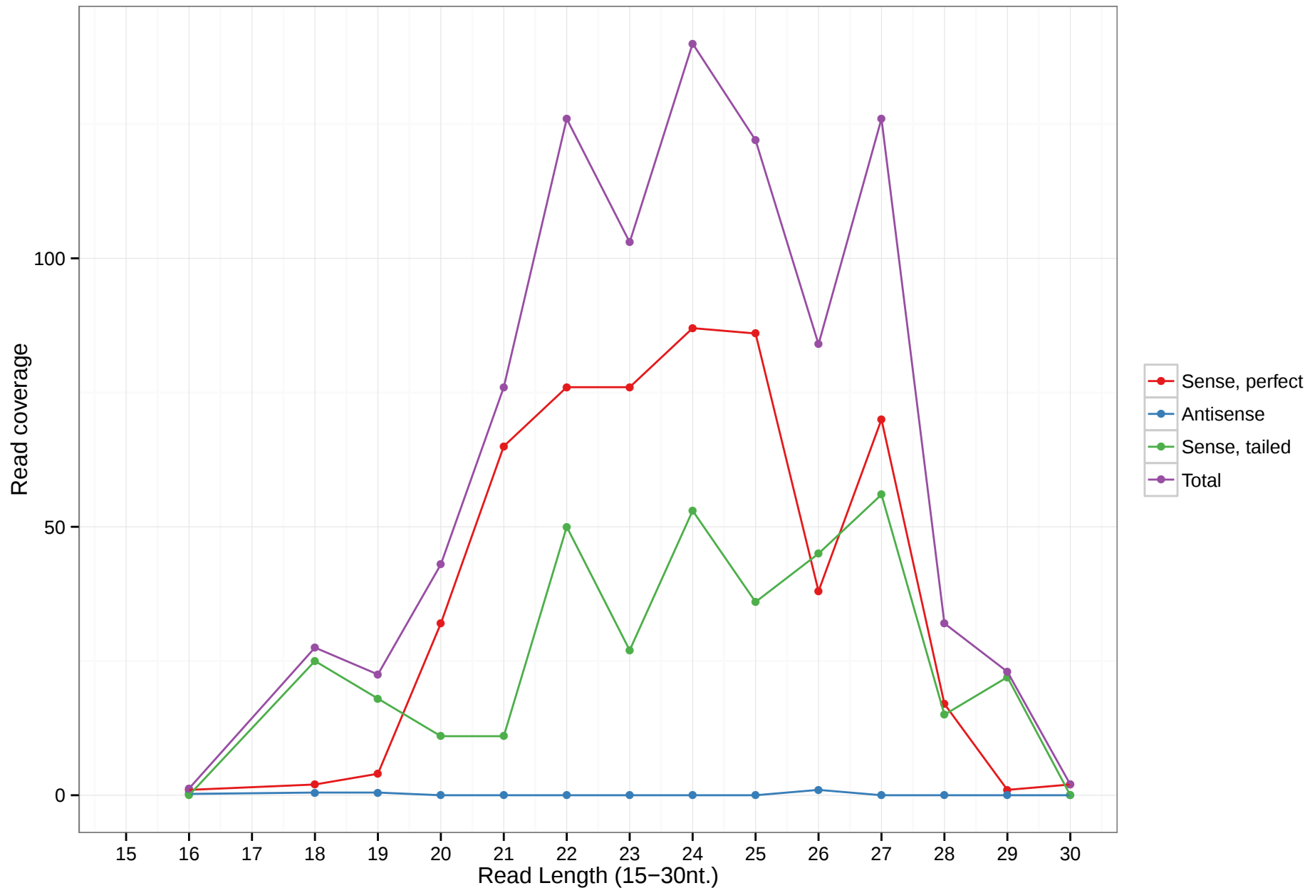
mmu-mir-7017
