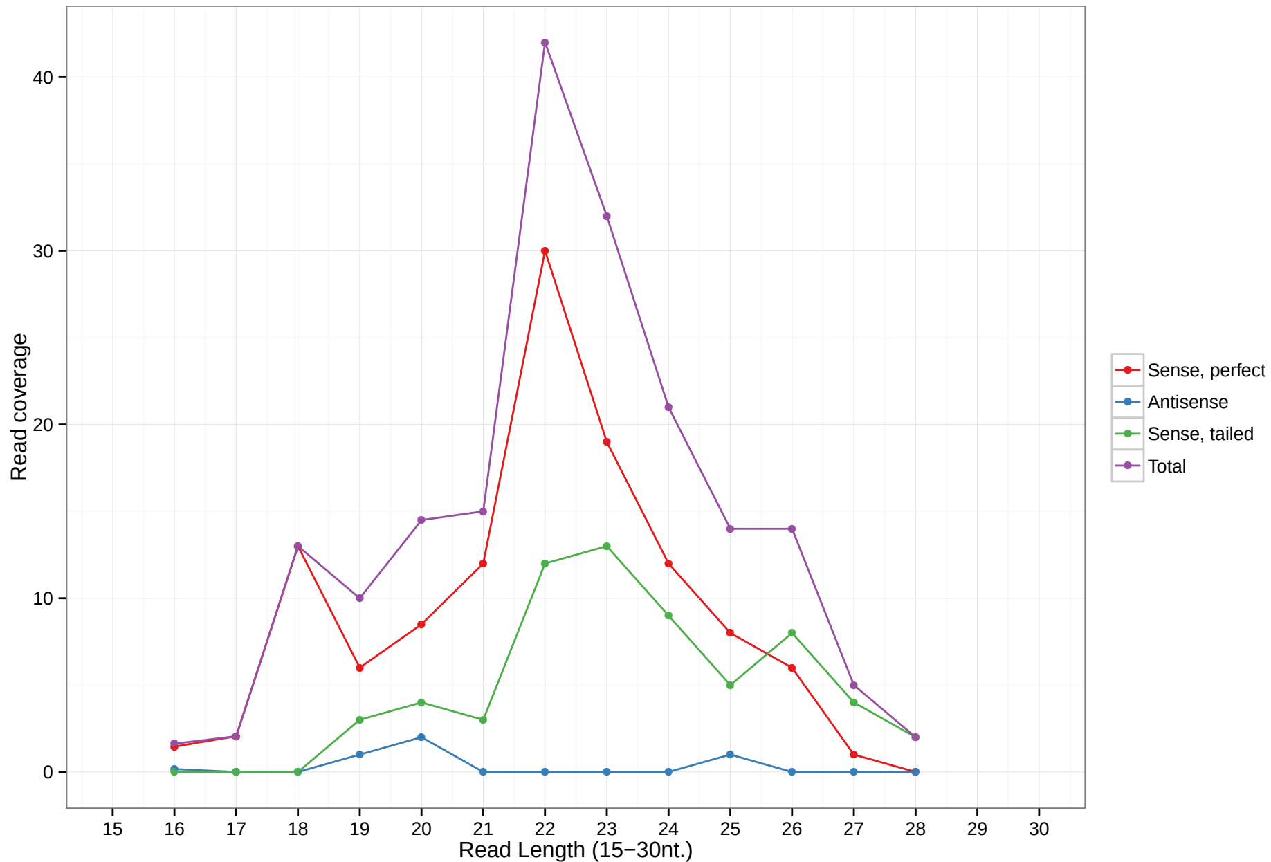
mmu-mir-7011
