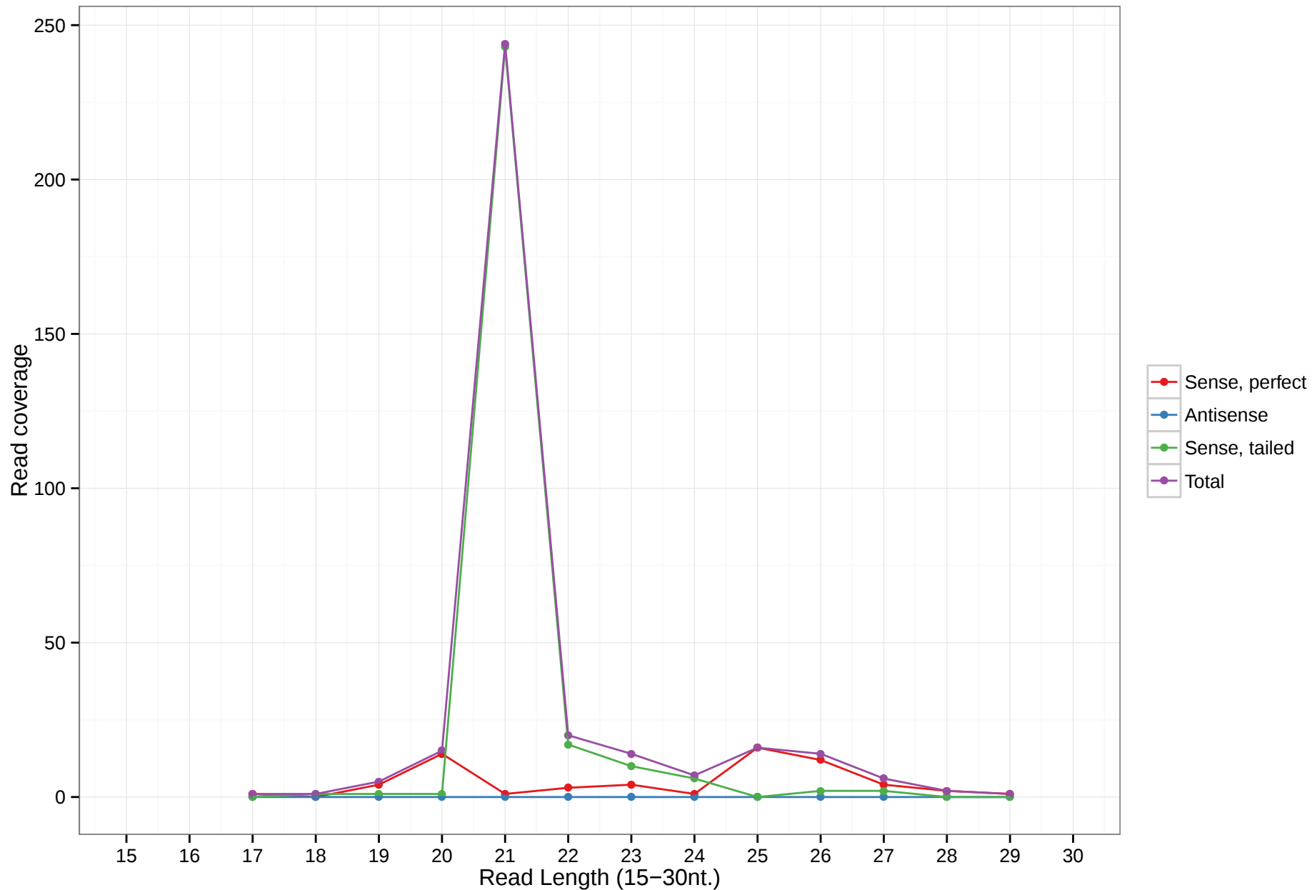
mmu-mir-7006
