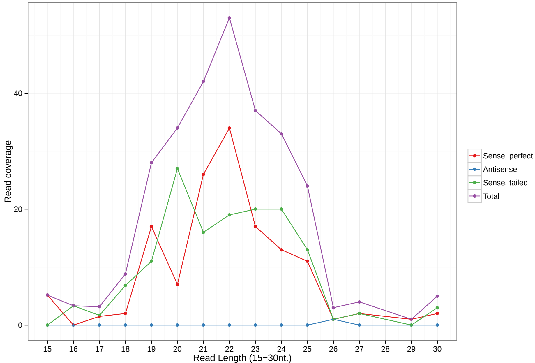
mmu-mir-7003
