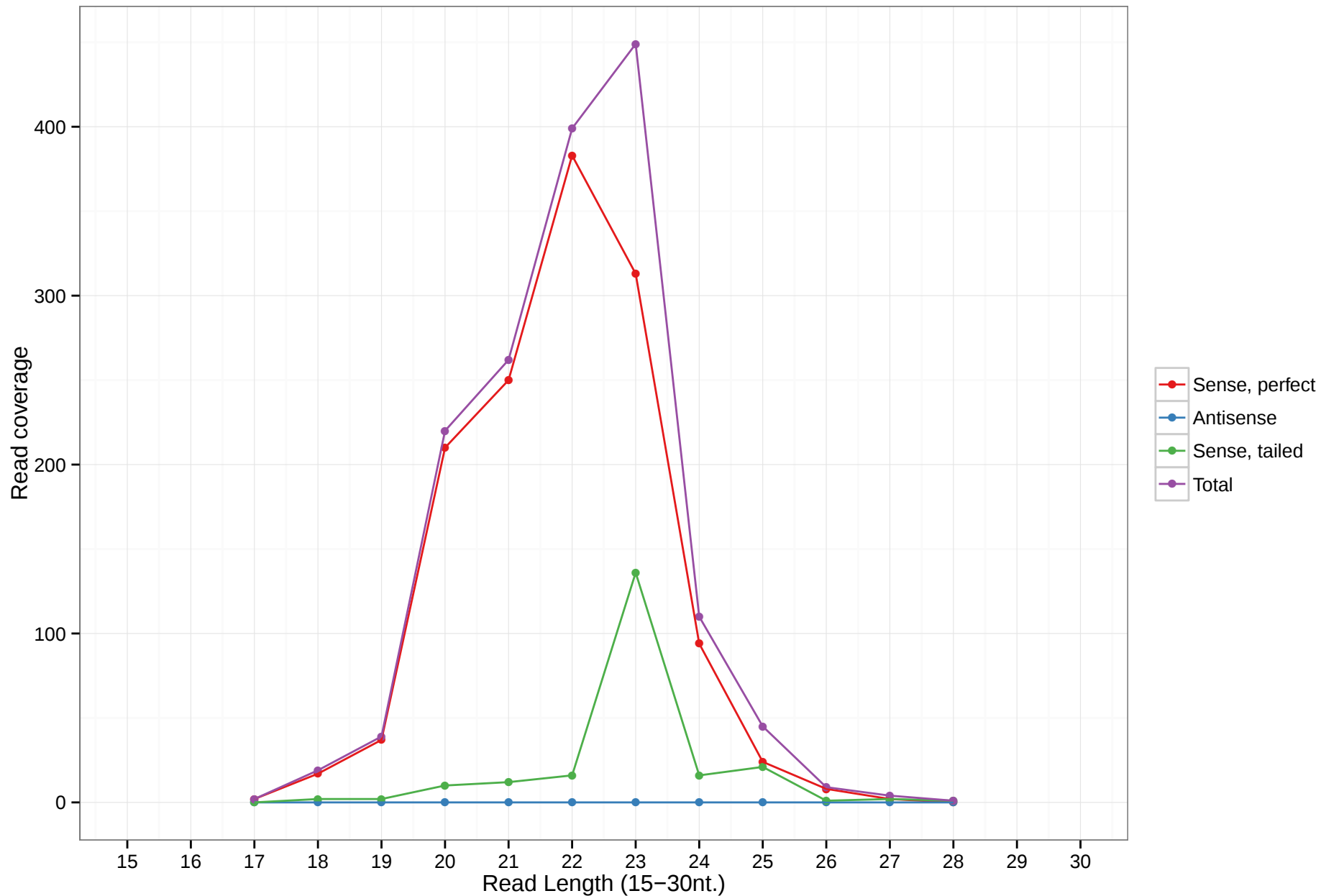
mmu-mir-3103
