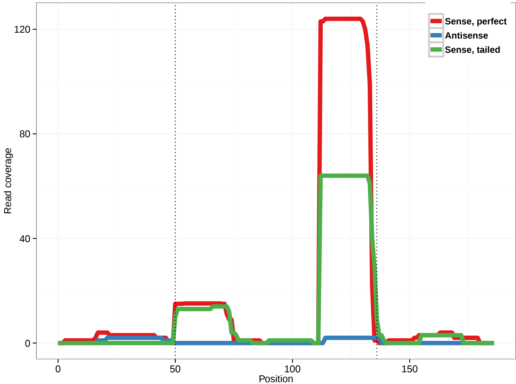
mmu-mir-7088
