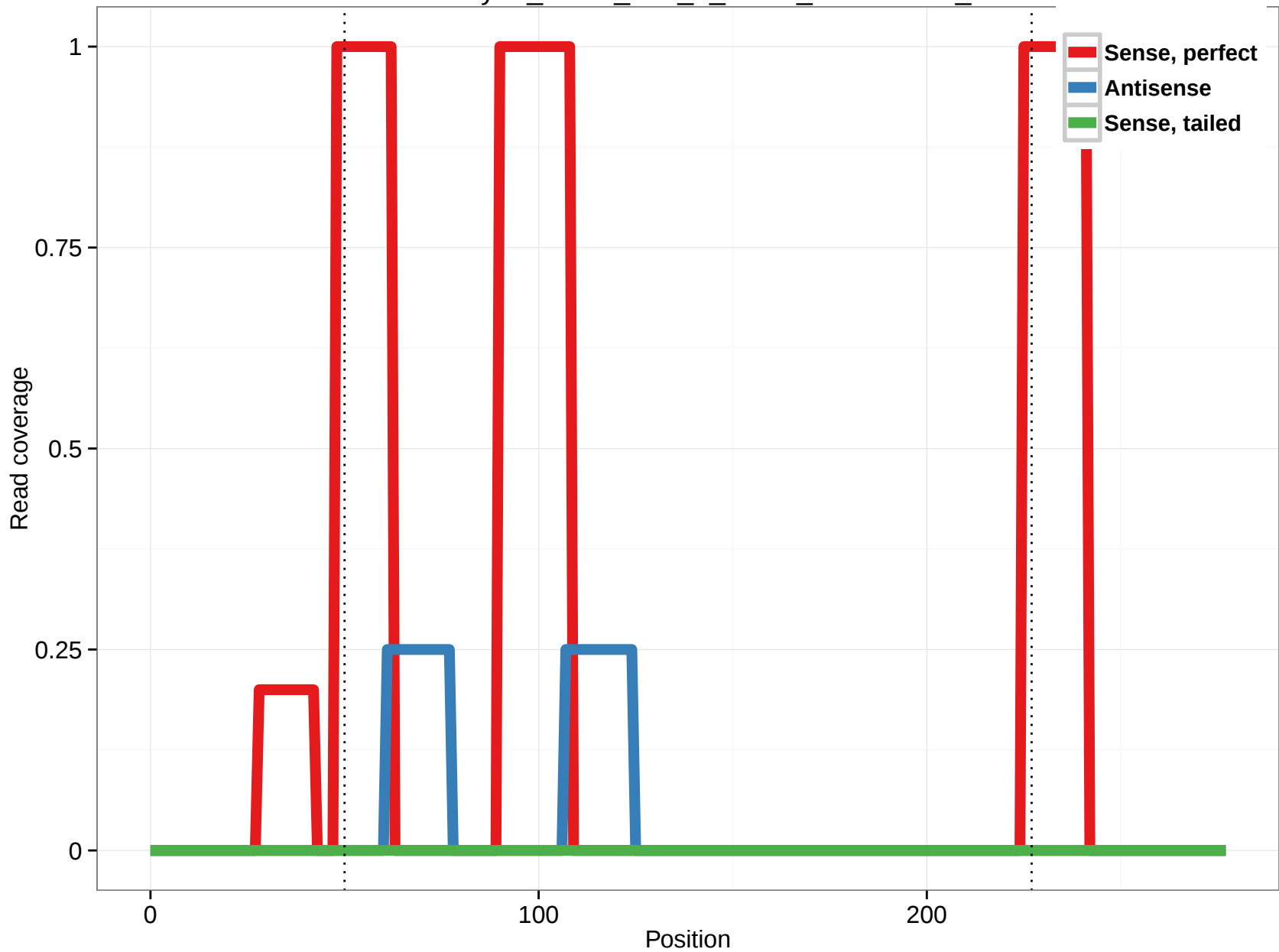
uc010tyt.1_intron_594_0_chr14_106356693_r
