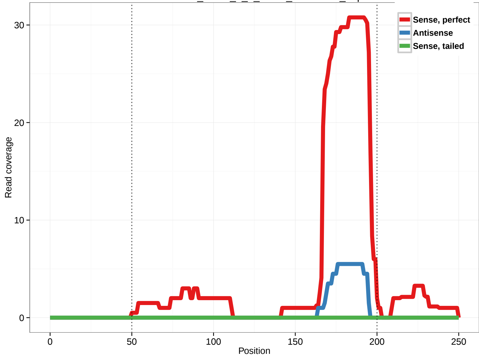
uc010tvk.1_intron_5_0_chr14_77932011_f.3p
