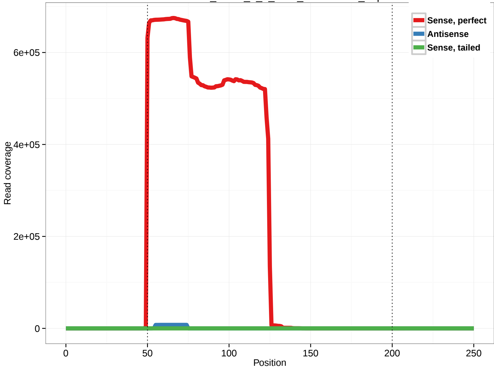
uc010nsf.1_intron_6_0_chrX_135961283_r.3p
