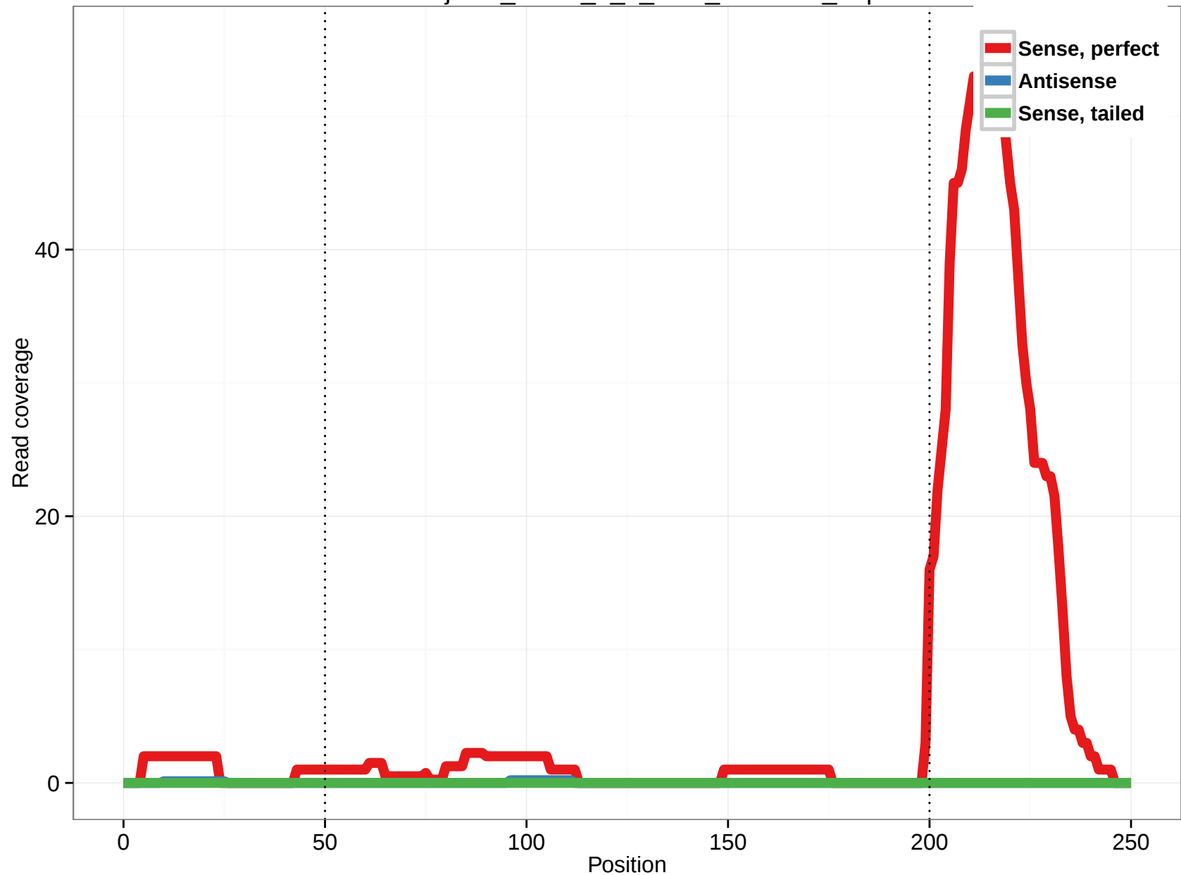
uc010jnz.2_intron_6_0_chr6_7895436_r.3p
