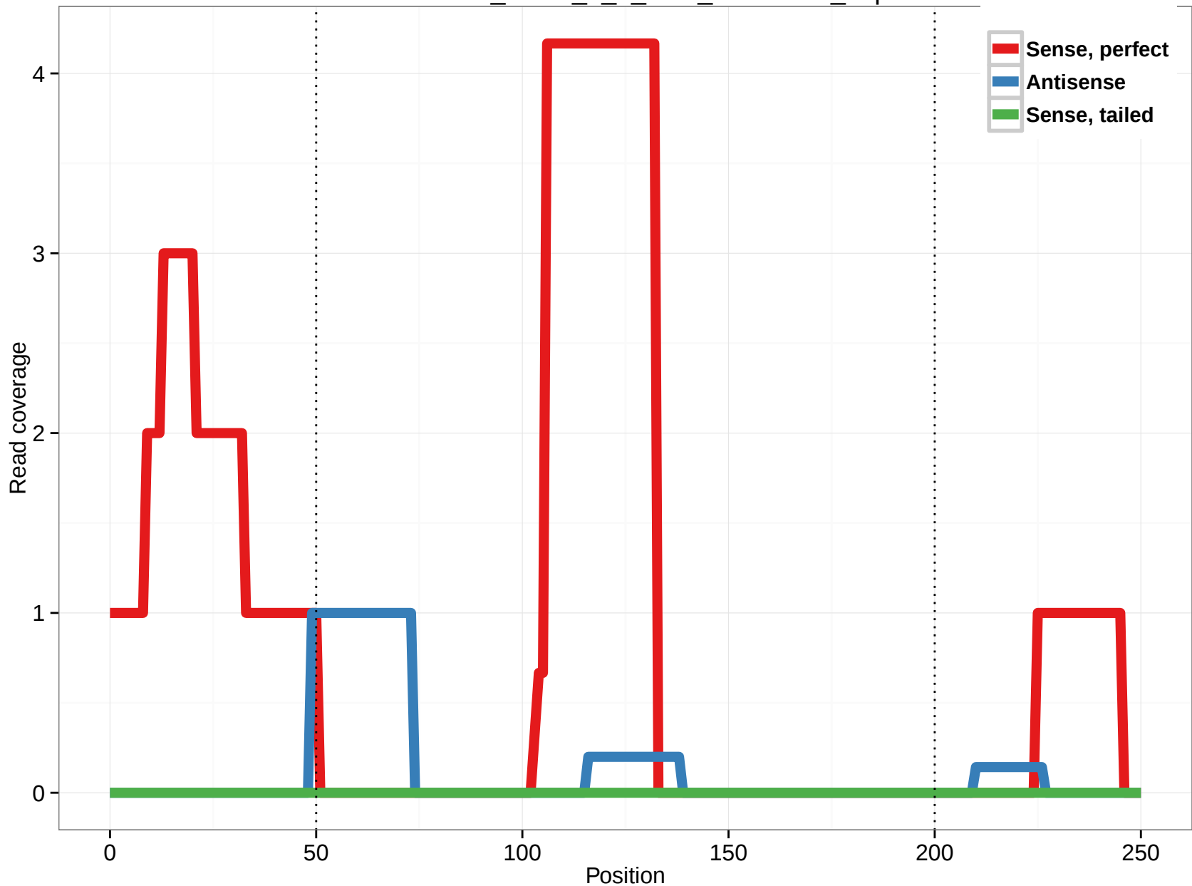
uc010ezf.2_intron_7_0_chr2_27858102_f.5p
