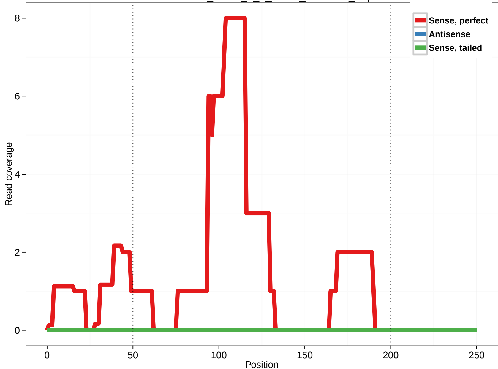
uc010ckn.1_intron_1_0_chr17_3831333_r.3p
