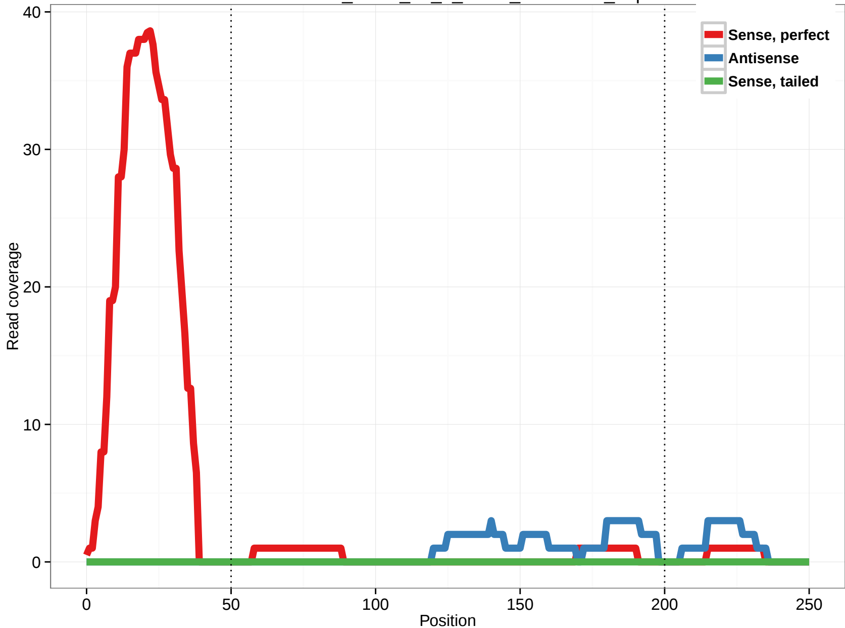
uc010auf.1_intron_13_0_chr14_92480922_r.5p
