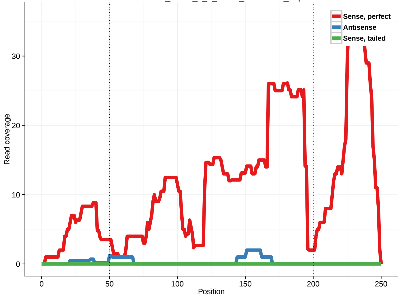
uc009znh.2_intron_6_0_chr12_54676663_f.3p
