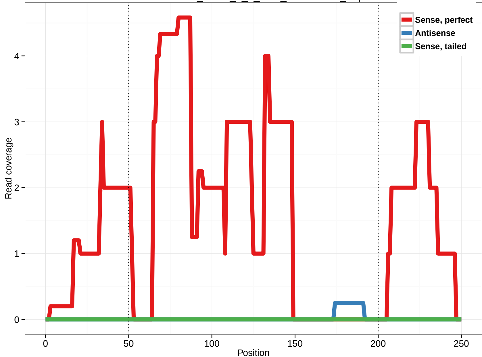
uc009wzt.1_intron_9_0_chr1_201342530_r.3p
