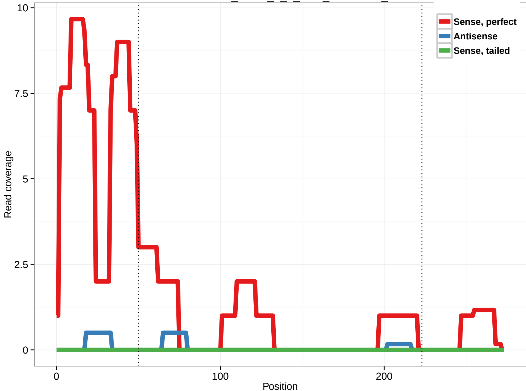
uc009wde.2_intron_5_0_chr1_92181952_r
