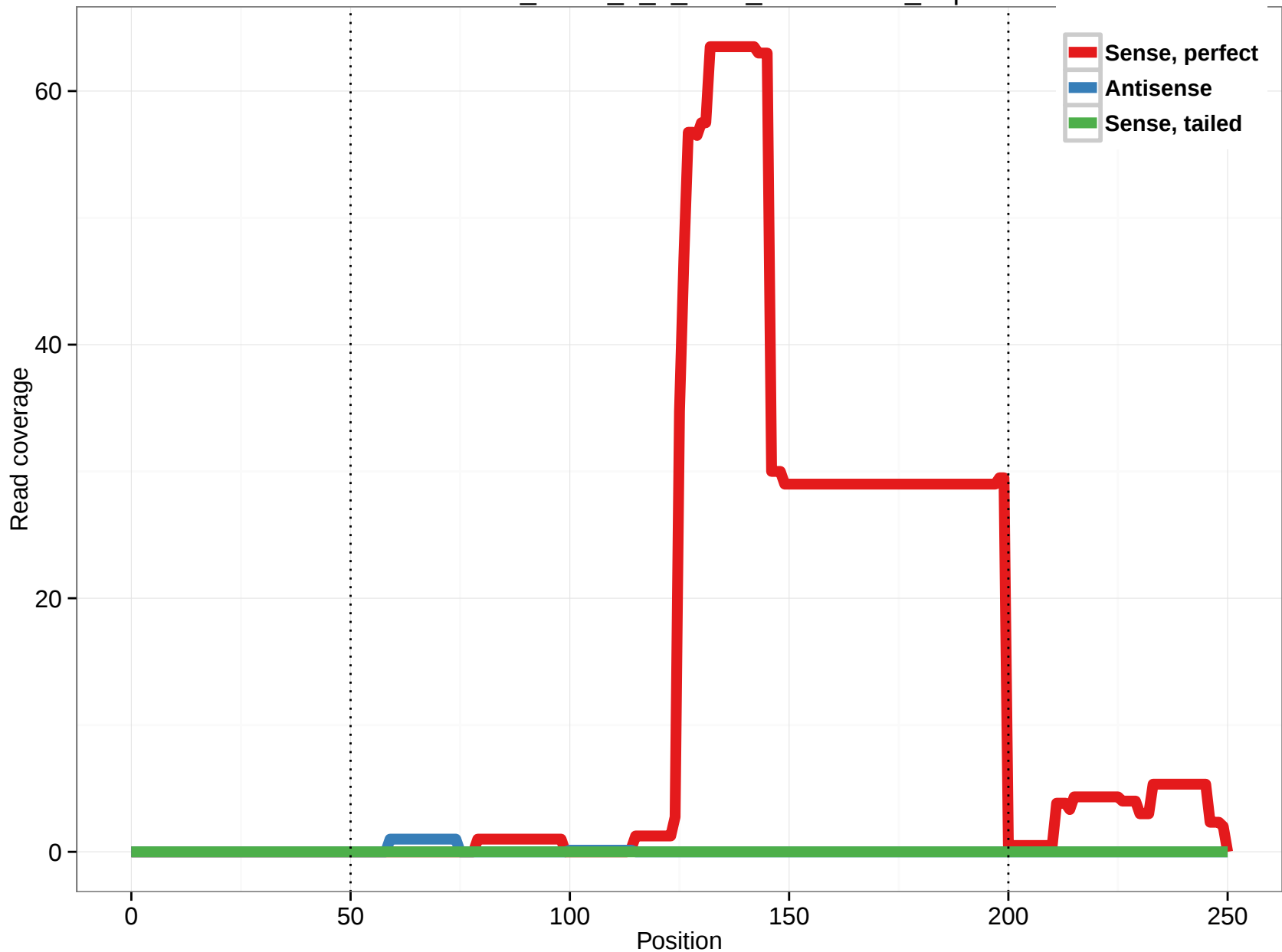
uc004flx.1_intron_7_0_chrX_153762712_r.3p
