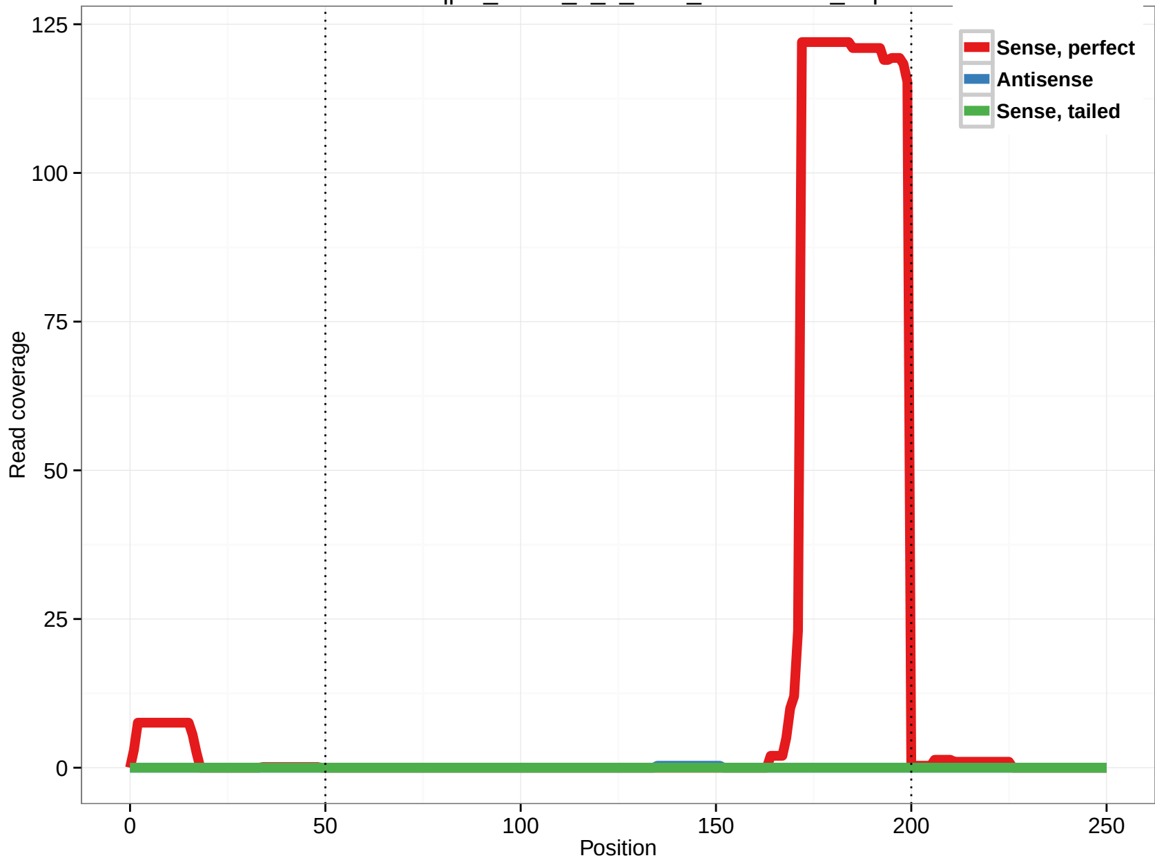
uc004eqp.2_intron_6_0_chrX_117695481_f.3p
