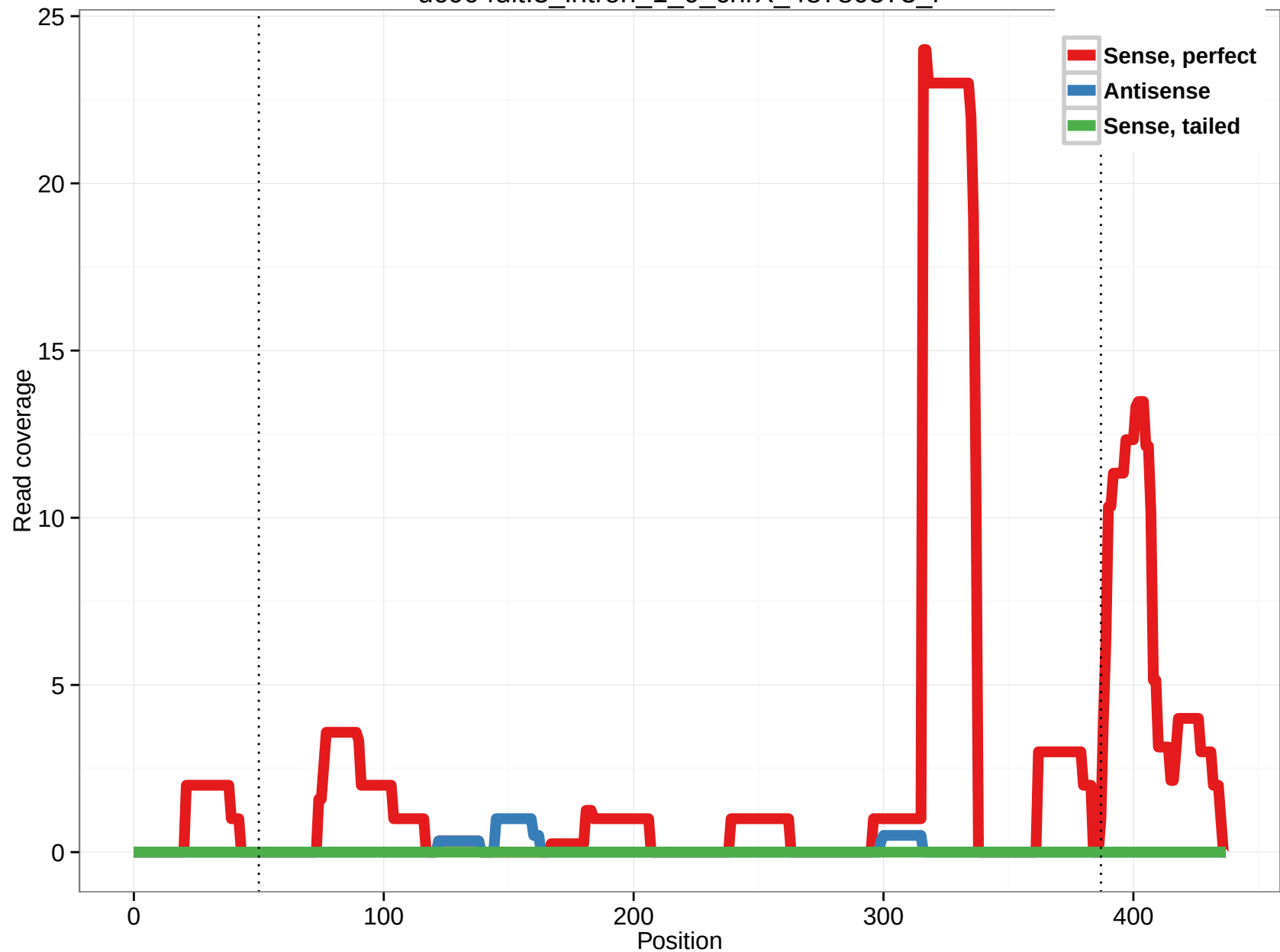
uc004dlt.3_intron_1_0_chrX_48780573_r
