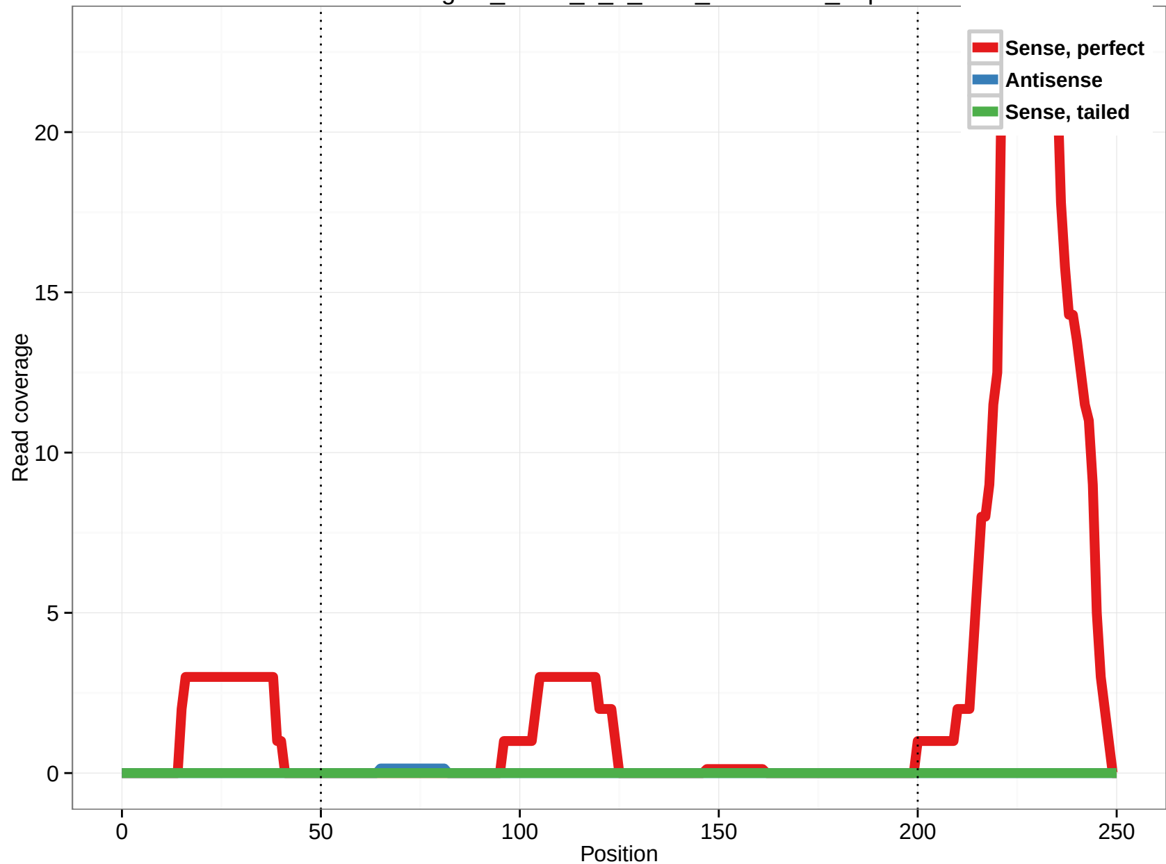
uc004dgz.1_intron_4_0_chrX_46949391_f.3p
