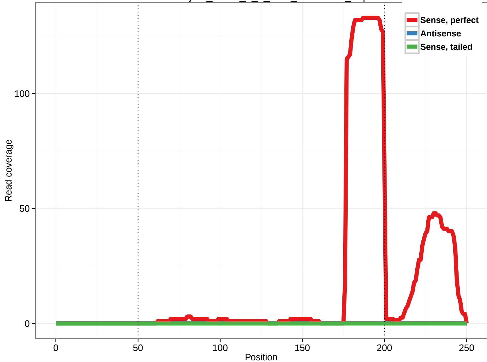
uc004aje.1_intron_1_0_chr9_75769498_f.3p
