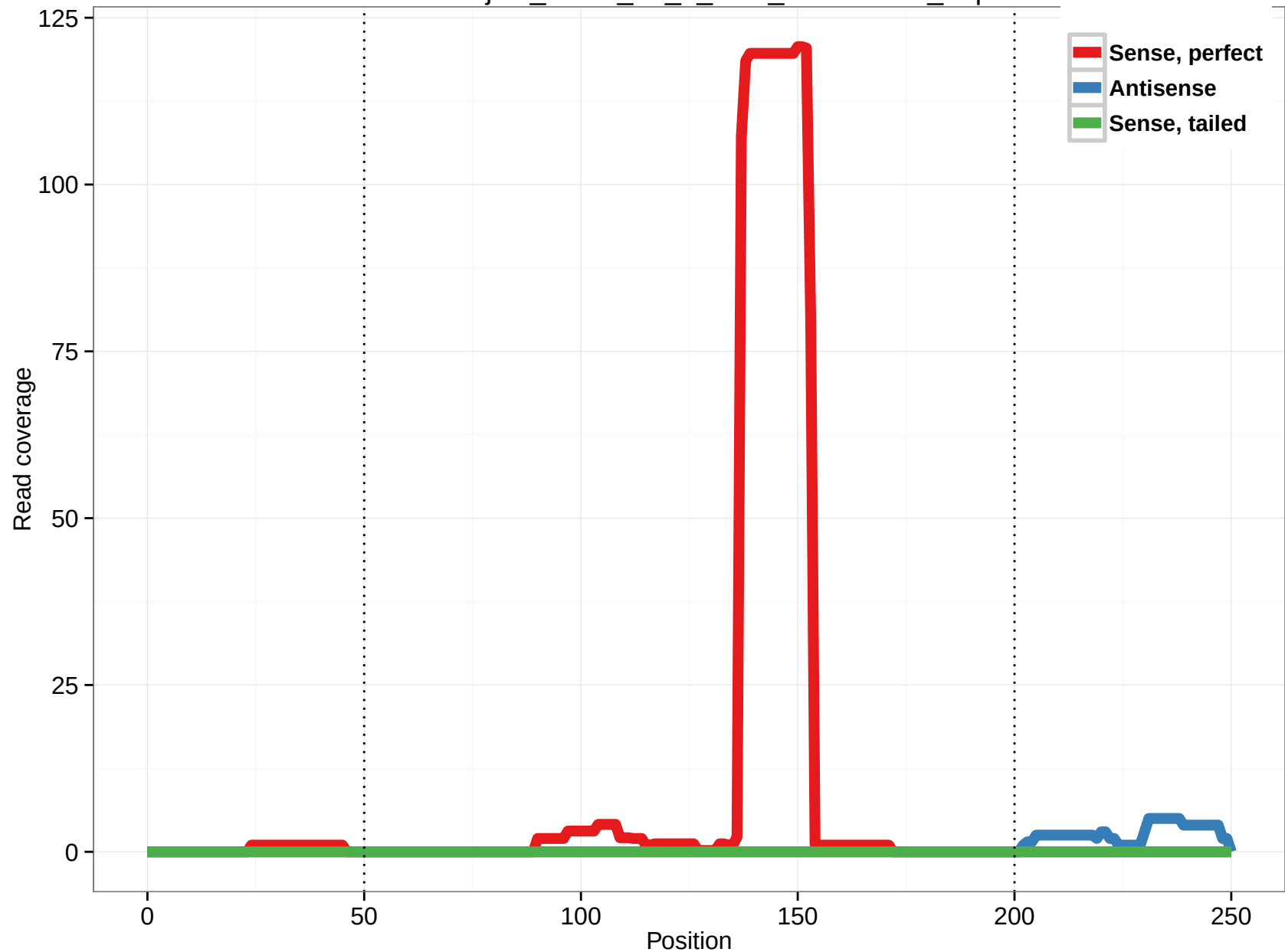
uc003wjs.2_intron_11_0_chr7_150942758_r.5p
