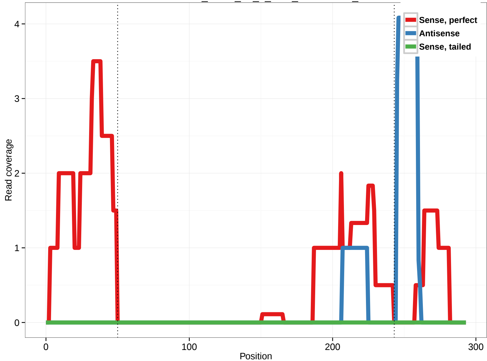
uc003wil.3_intron_11_0_chr7_150737722_f
