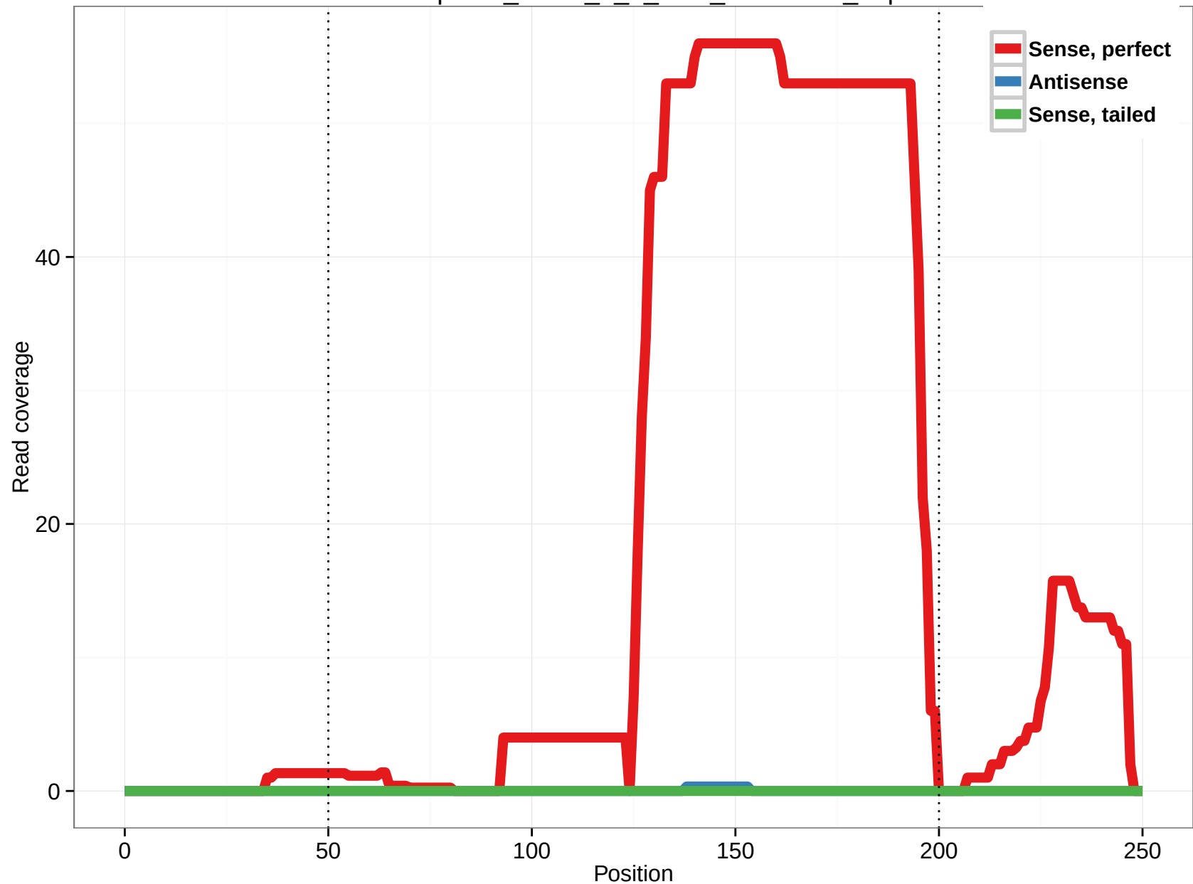
uc003pan.1_intron_4_0_chr6_52134025_r.3p
