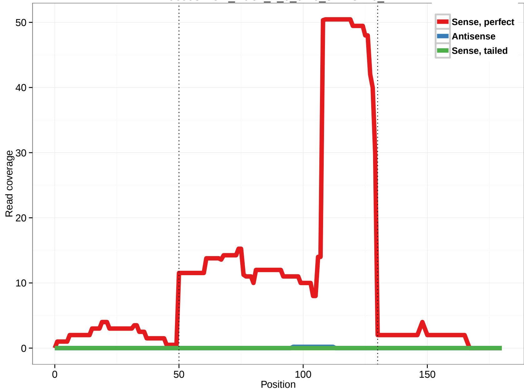
uc003nxe.2_intron_7_0_chr6_31748716_r
