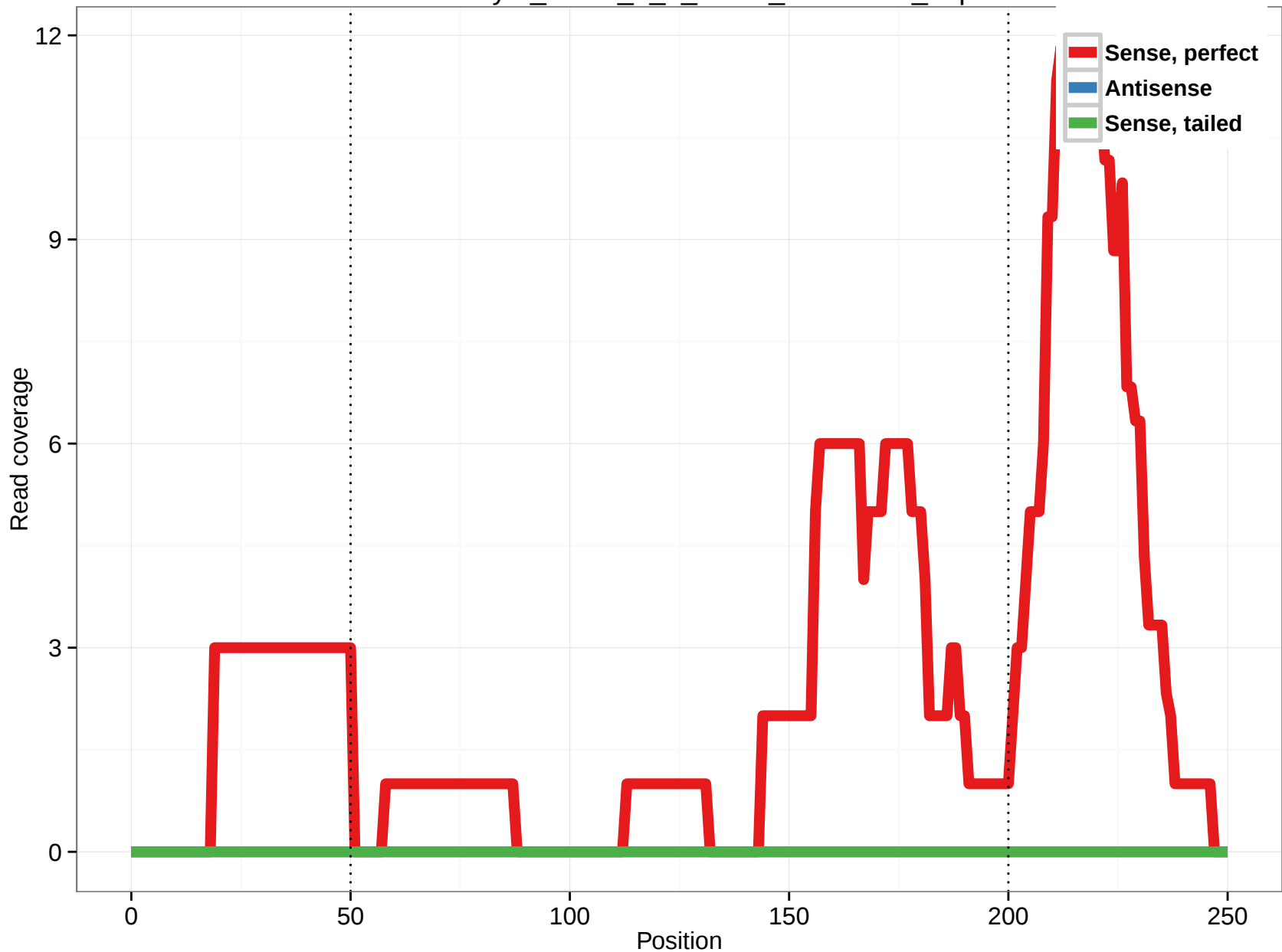
uc003bky.1_intron_4_0_chr22_50853119_f.3p
