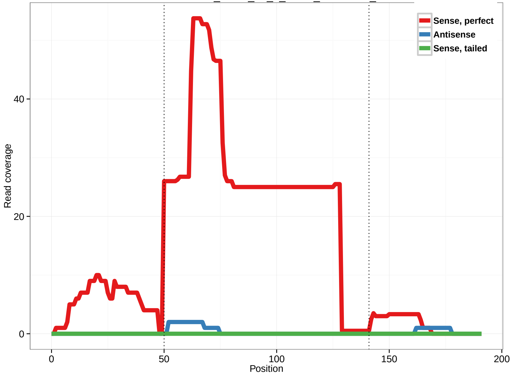
uc003azw.2_intron_18_0_chr22_41751867_f
