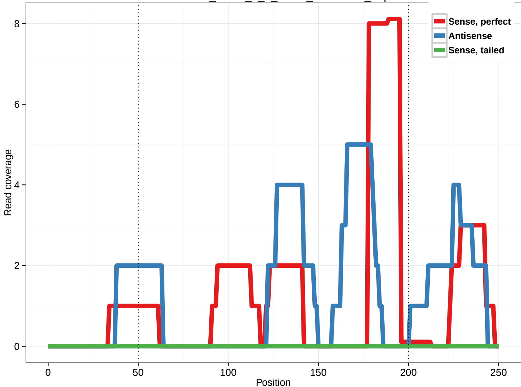
uc002zlt.2_intron_6_0_chr22_17129539_f.3p
