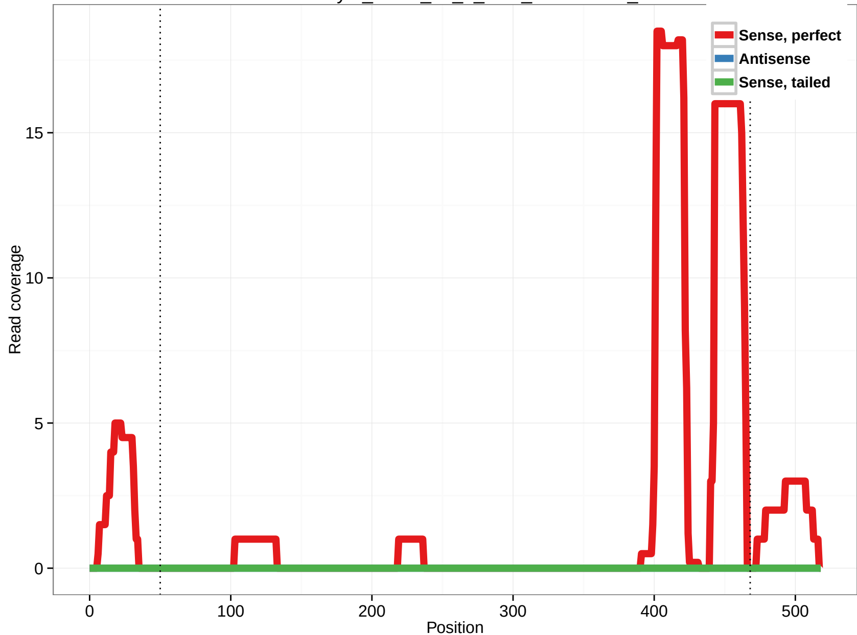
uc002vzy.2_intron_31_0_chr2_241708626_r
