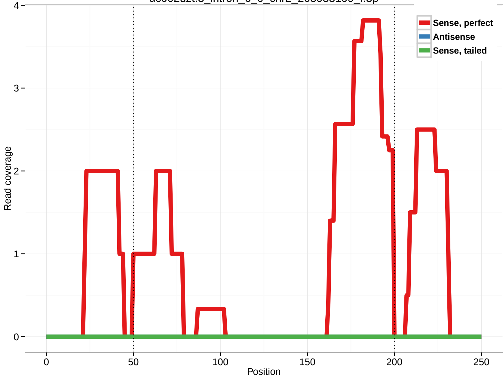
uc002uzt.3_intron_6_0_chr2_203933199_f.3p
