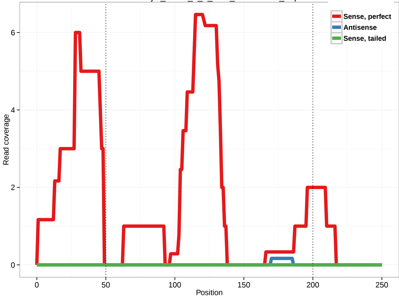
uc002toj.1_intron_7_0_chr2_128081818_r.5p
