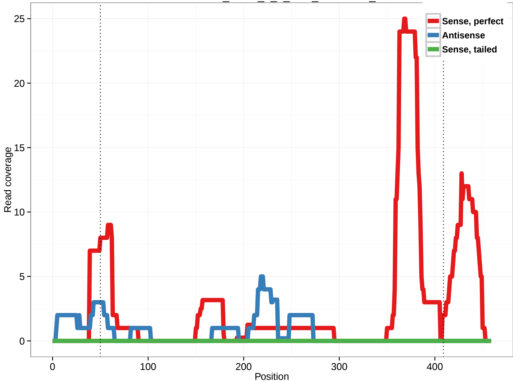
uc002rzw.3_intron_4_0_chr2_58390210_r
