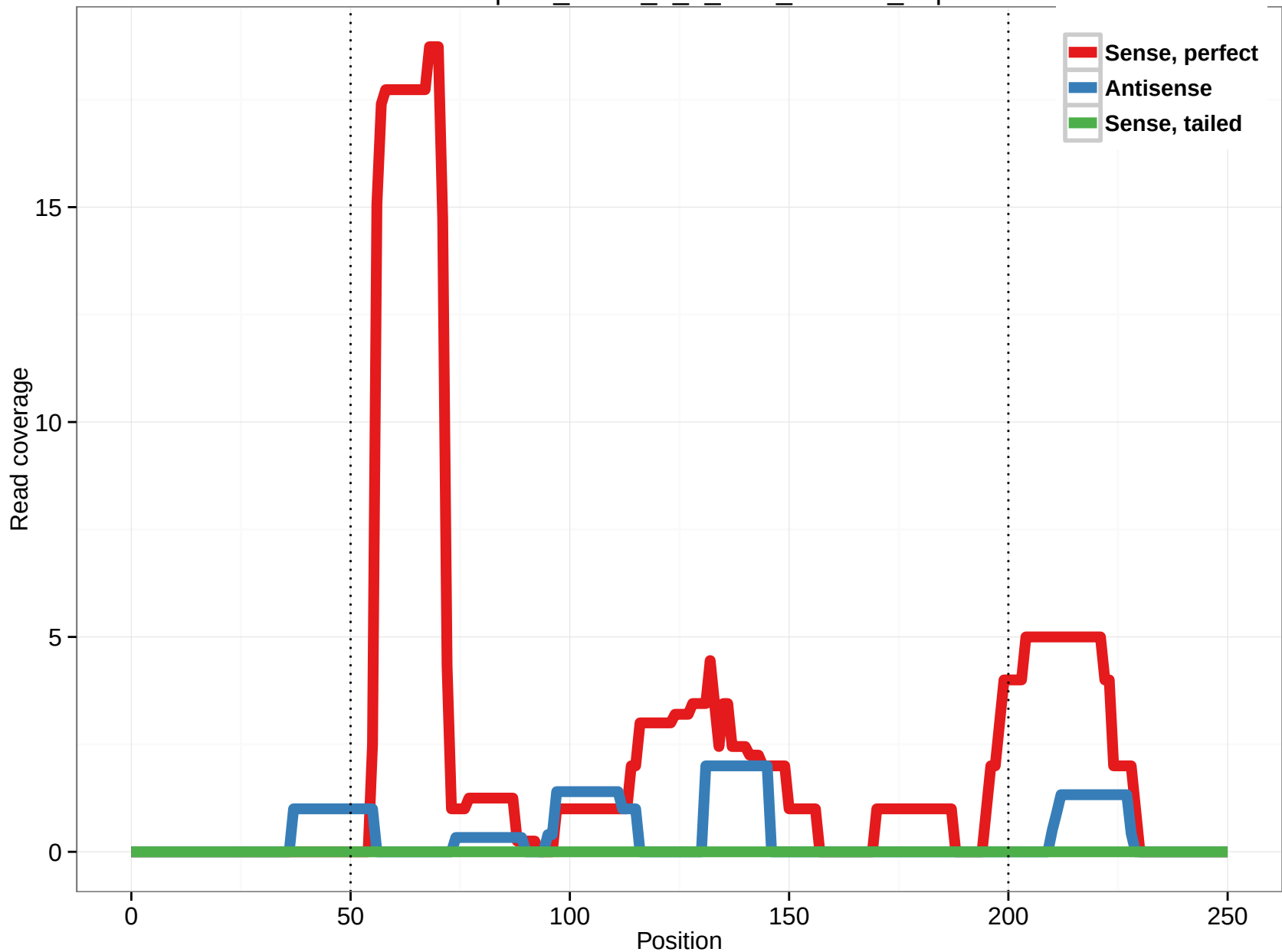
uc002qvz.2_intron_8_0_chr2_253116_r.5p
