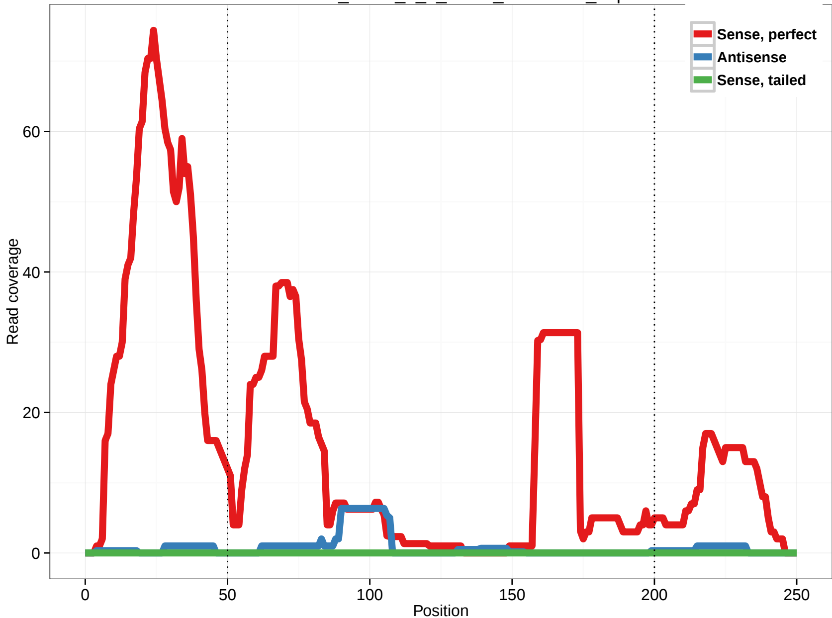
uc002lis.2_intron_0_0_chr18_60382770_f.5p
