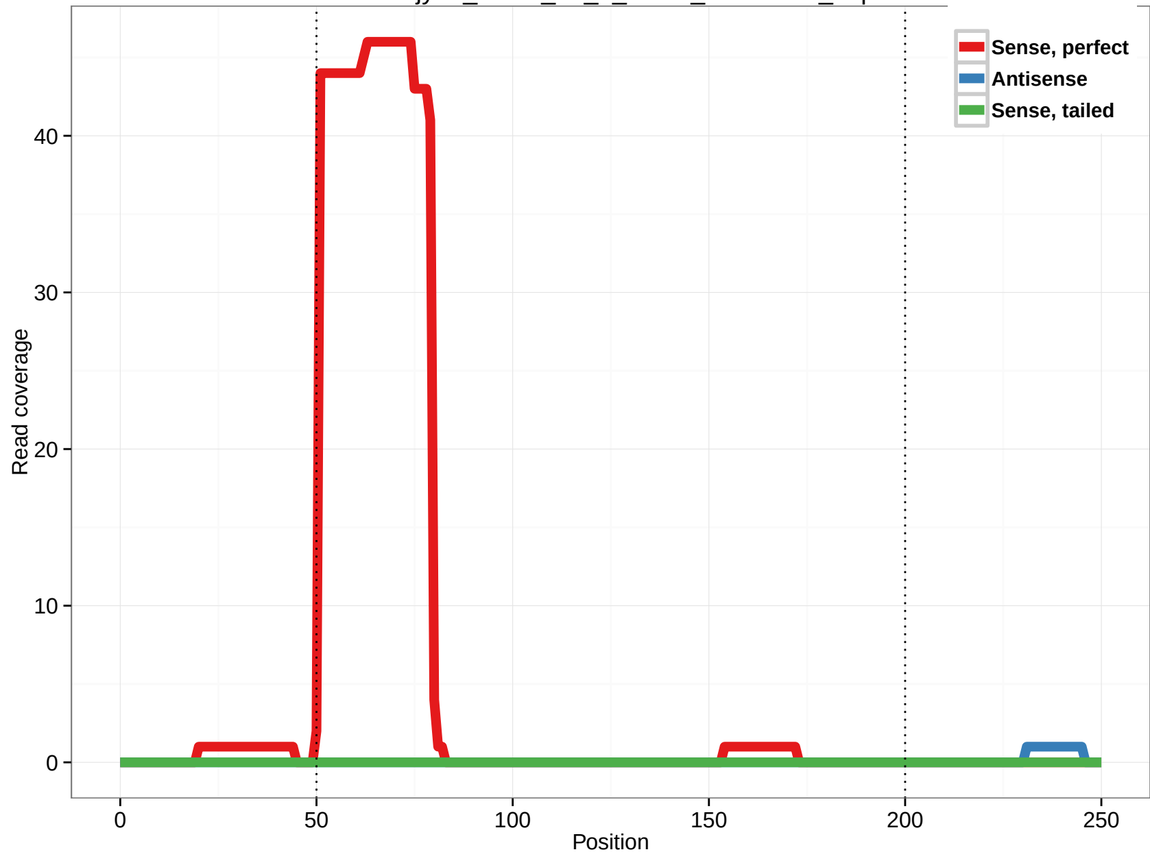
uc002jyt.1_intron_21_0_chr17_78896628_f.3p
