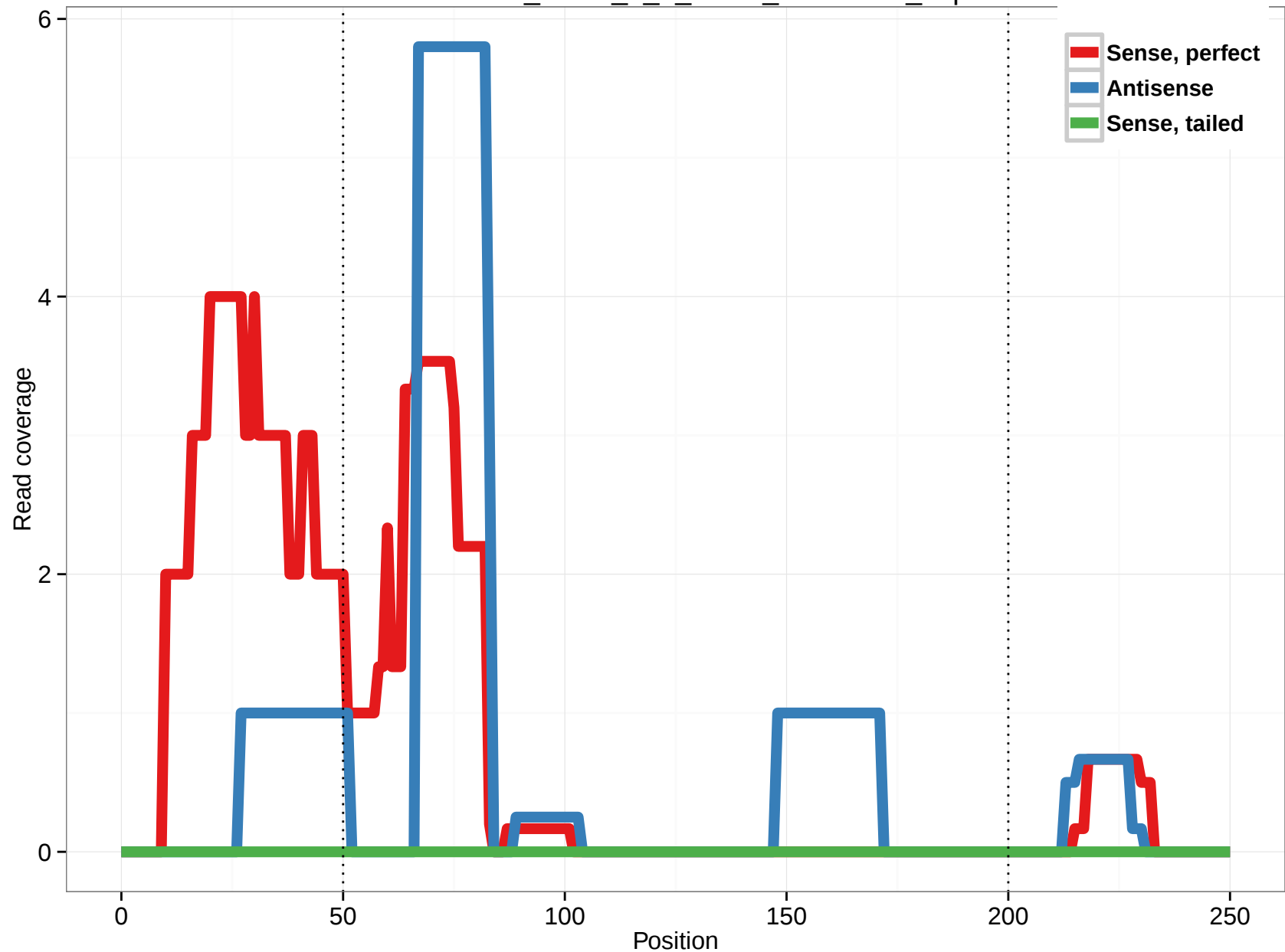
uc002hhr.2_intron_0_0_chr17_31255256_f.5p
