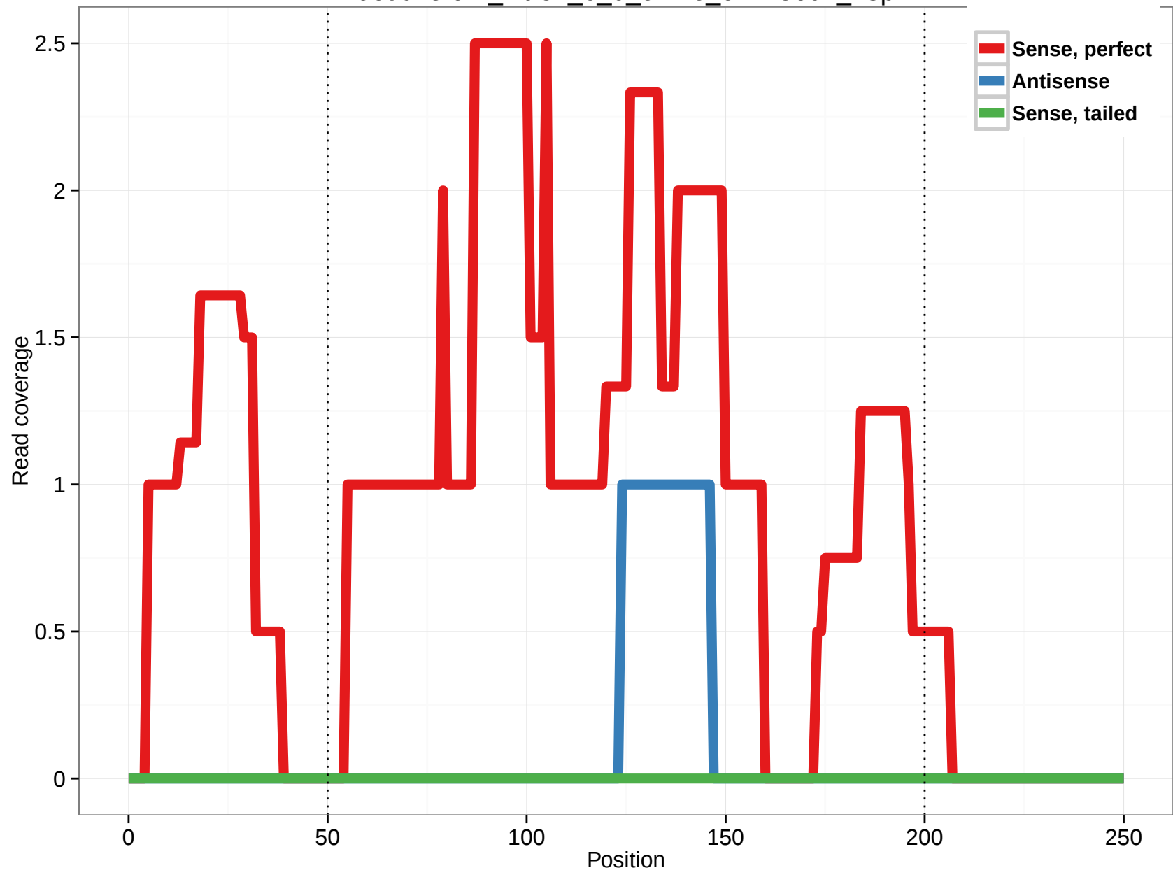
uc002eru.2_intron_6_0_chr16_67215601_r.3p
