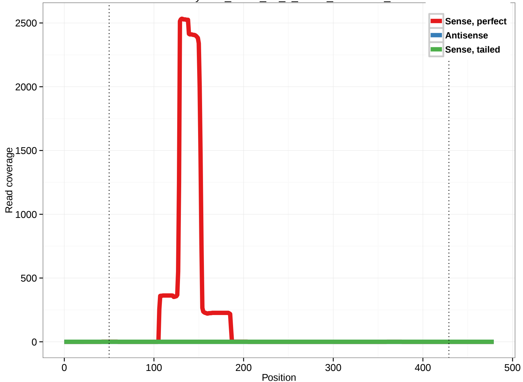
uc001yzw.1_intron_11_0_chr15_25477479_f
