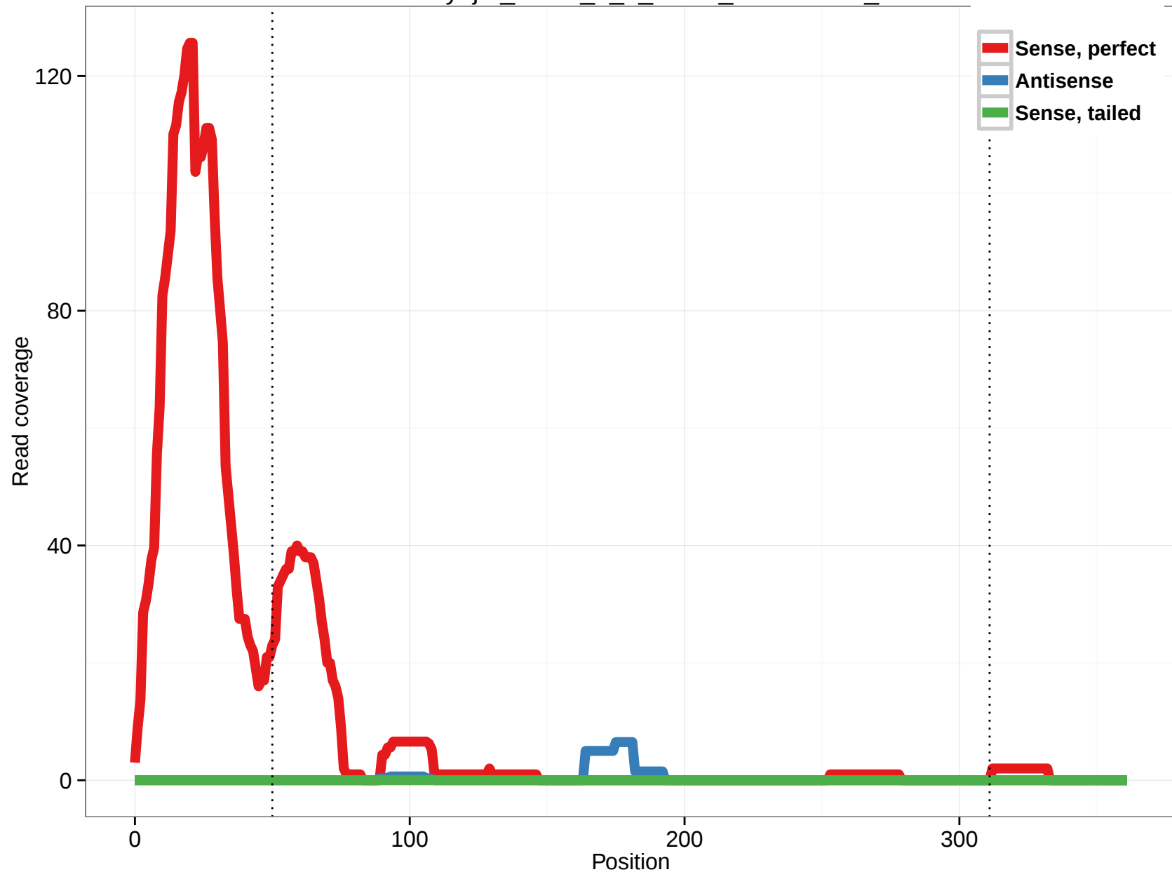
uc001yoj.3_intron_3_0_chr14_104387546_r
