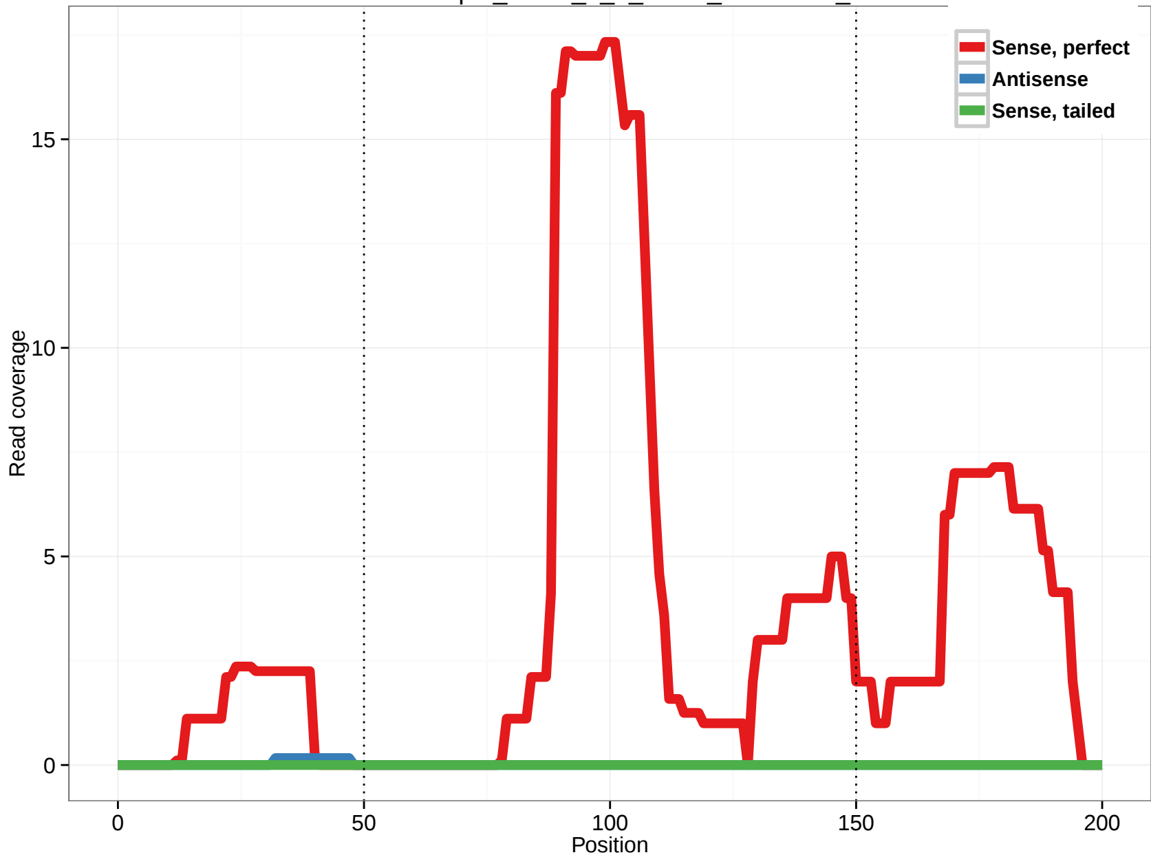
uc001vzp.2_intron_8_0_chr14_21546432_f
