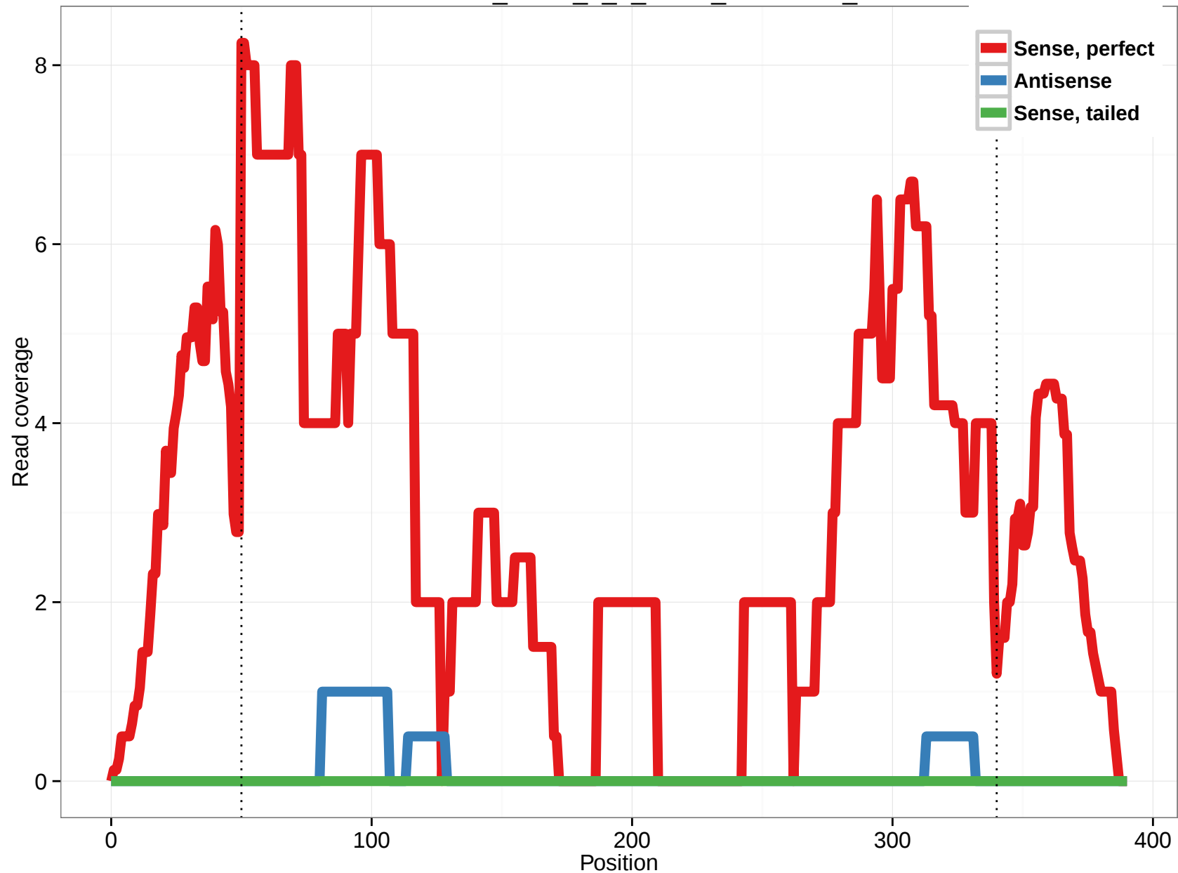
uc001sfl.2_intron_8_0_chr12_54677752_f
