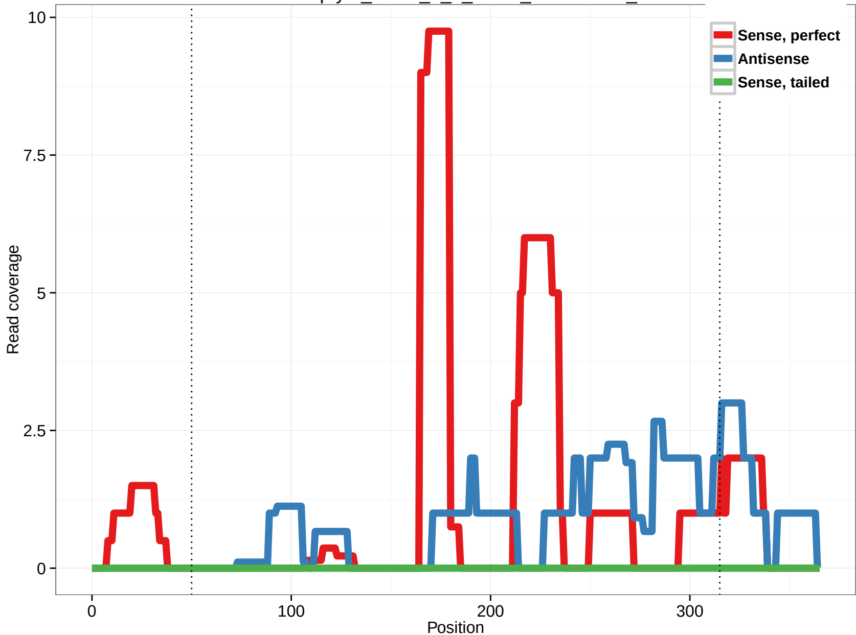
uc001pty.1_intron_4_0_chr11_118530191_r
