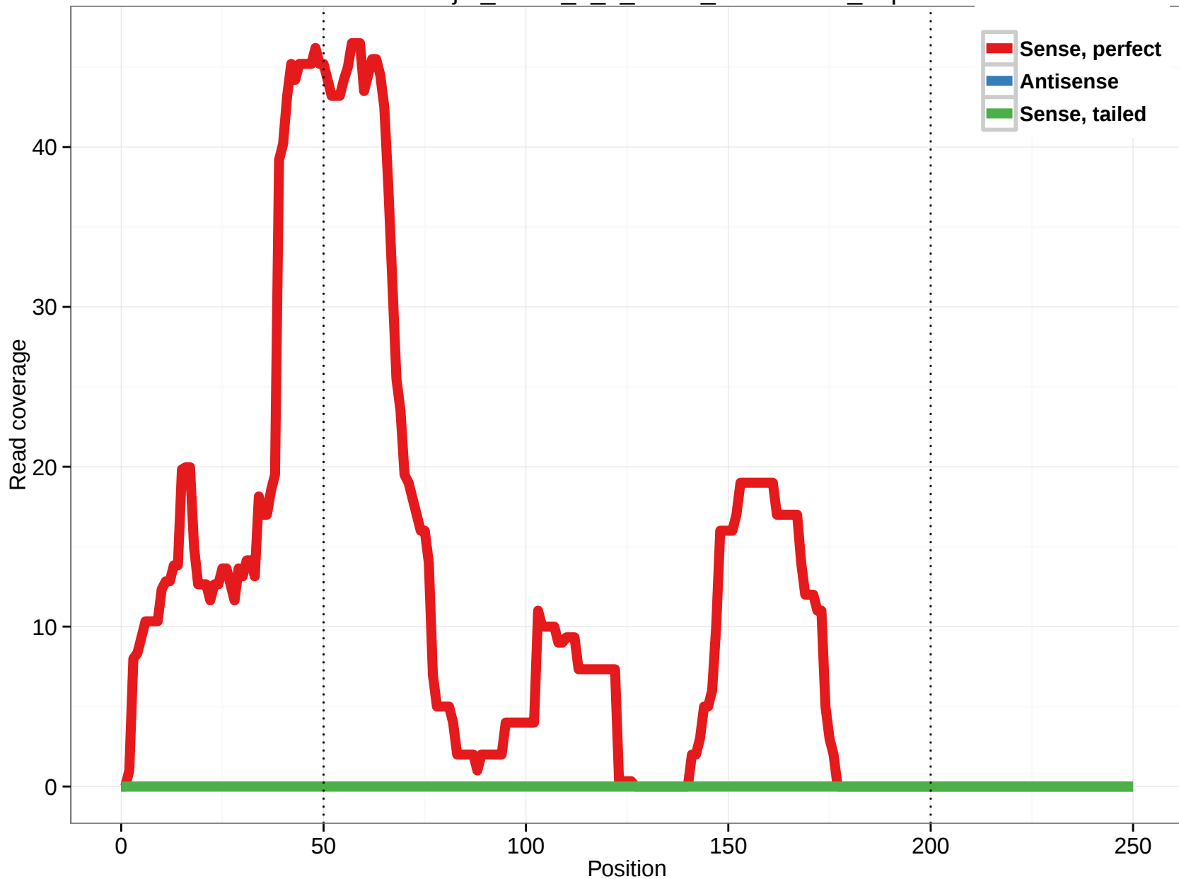
uc001kwj.2_intron_4_0_chr10_104622690_f.5p
