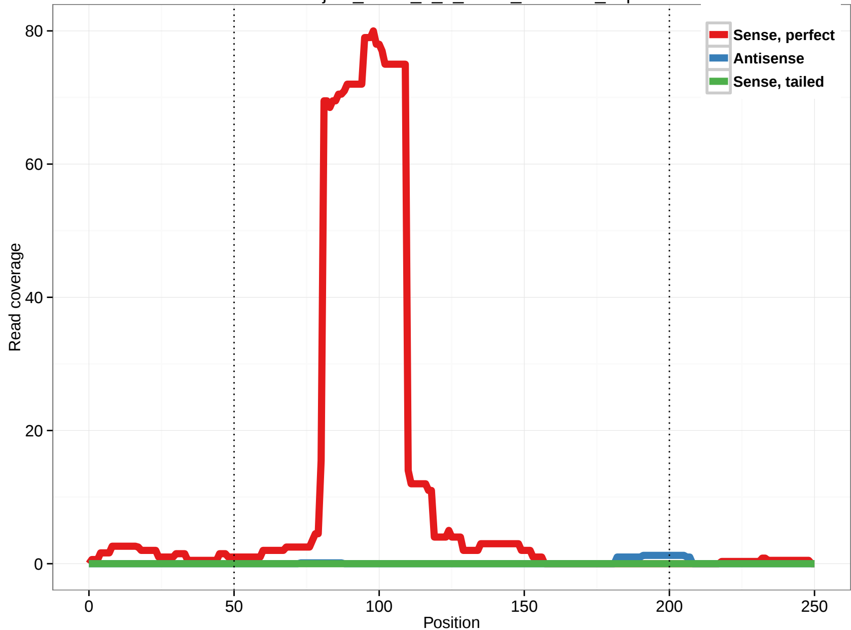
uc001ijd.2_intron_9_0_chr10_6263709_f.3p
