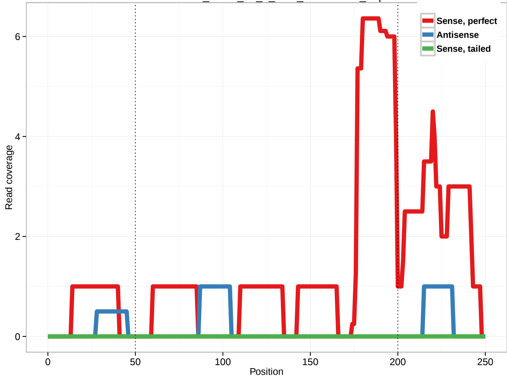
uc001ffw.2_intron_10_0_chr1_154941925_r.3p
