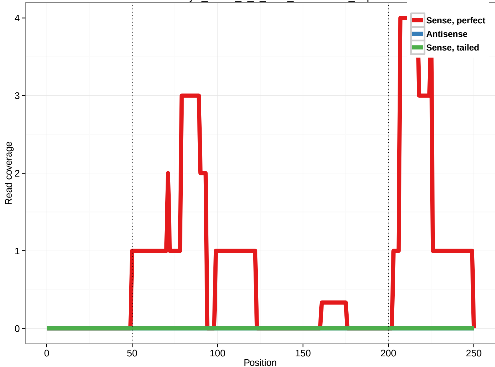
uc001eoj.2_intron_4_0_chr1_145682095_f.3p
