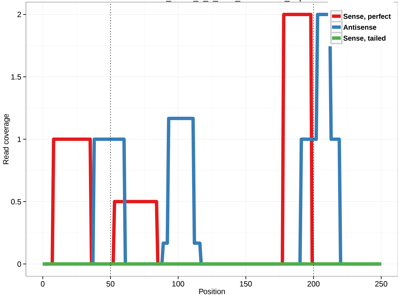
uc001edh.3_intron_7_0_chr1_114161229_f.5p
