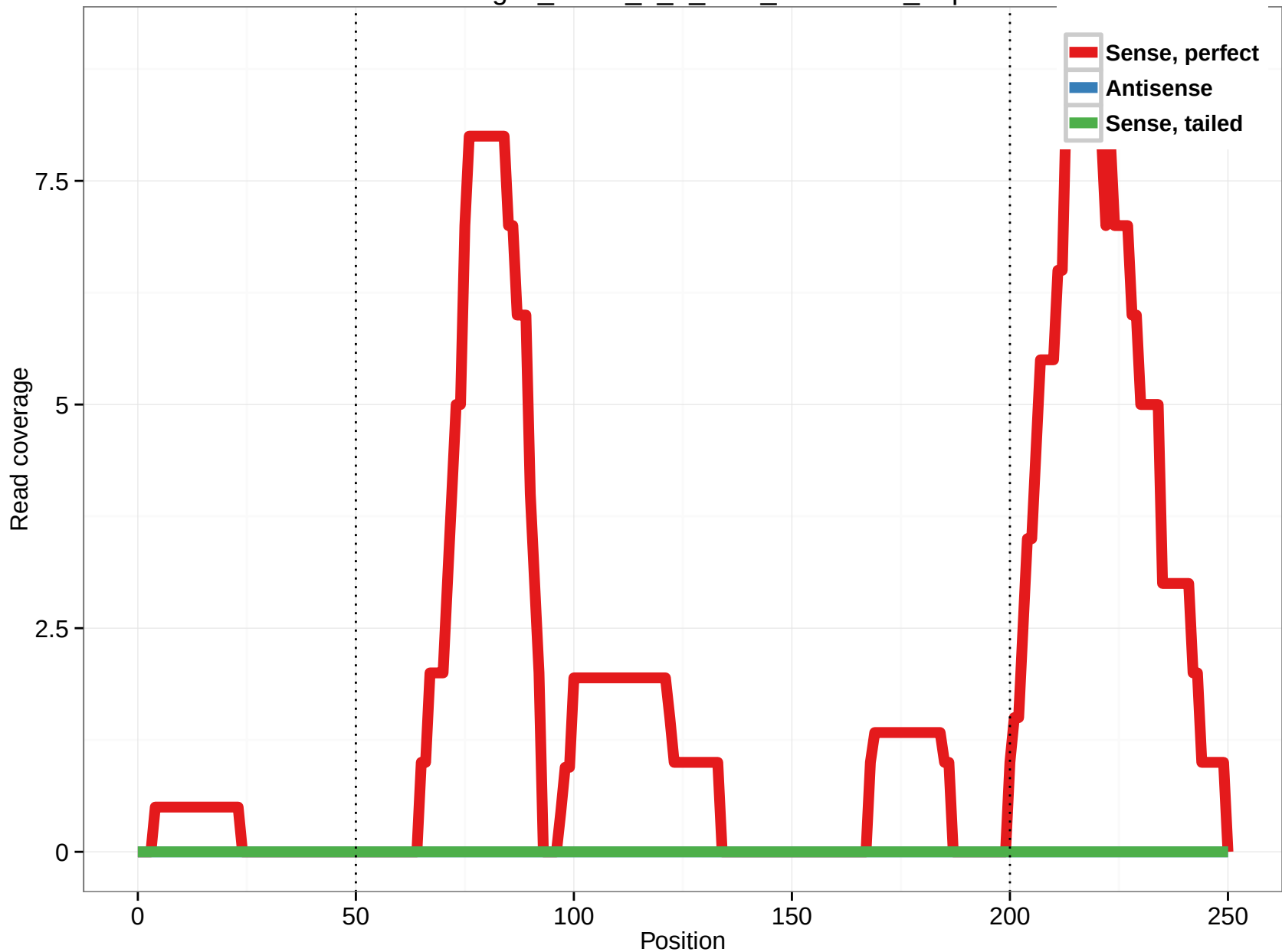
uc001dgl.2_intron_1_0_chr1_75172679_r.3p
